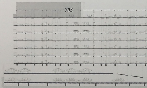
Corte Esquemático
