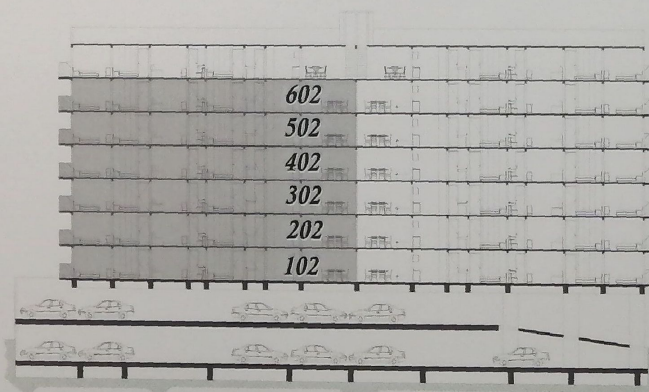
Corte Esquemático
