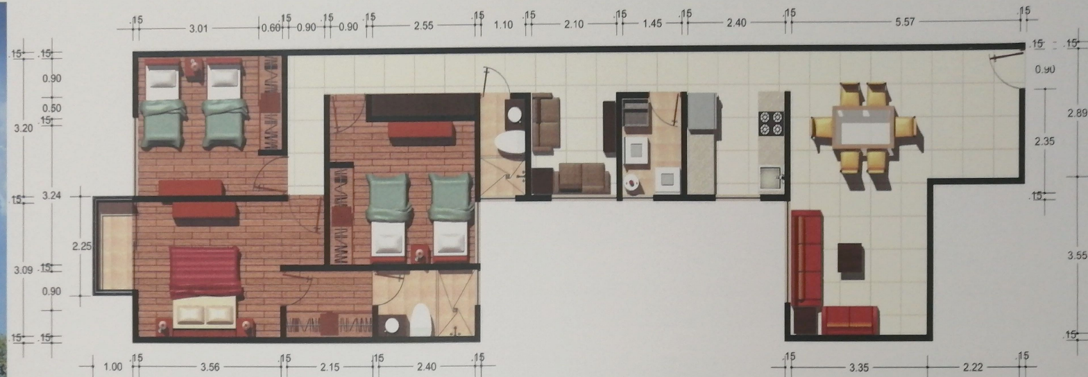
Planta Arquitectónica
