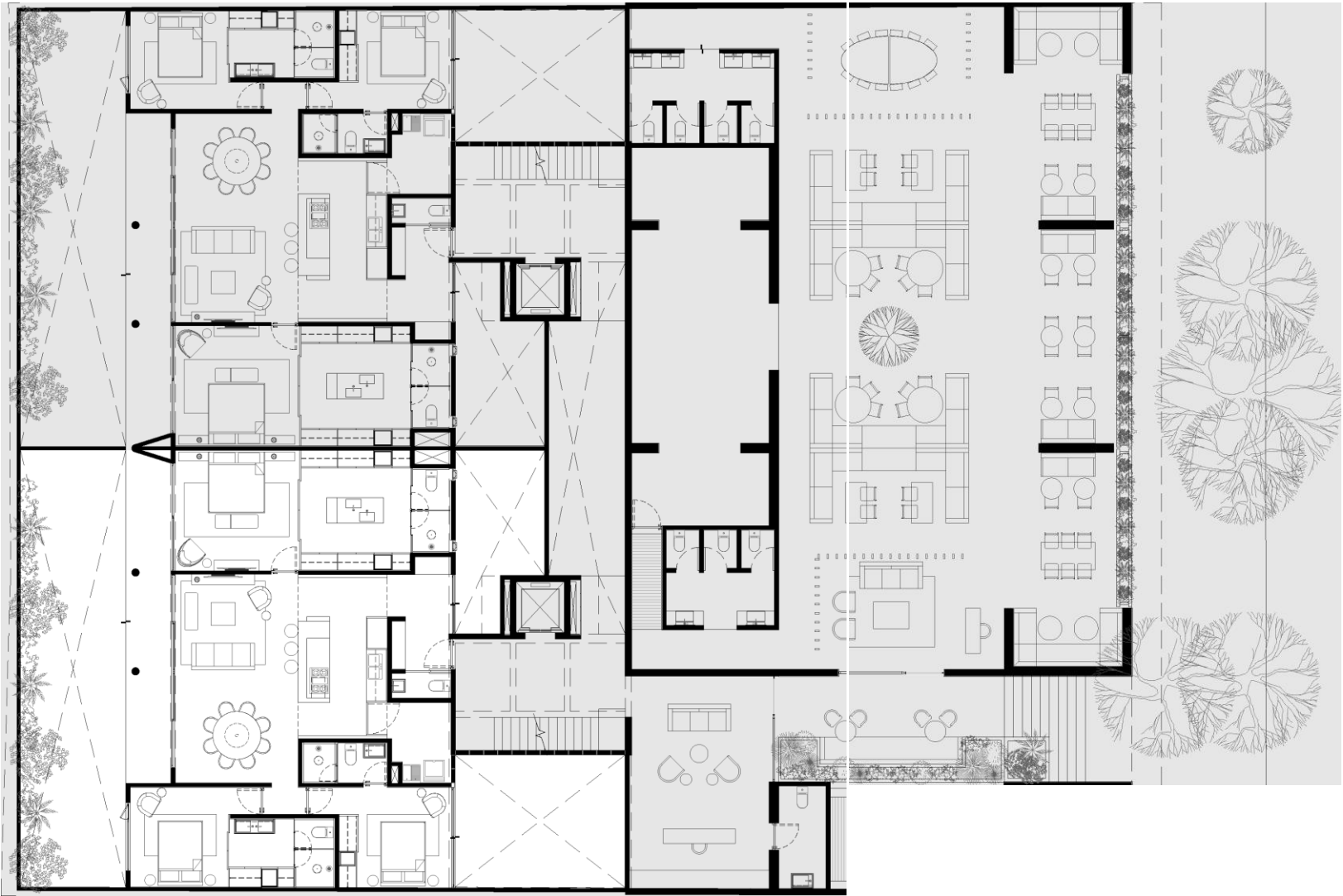
PRIMER NIVEL
