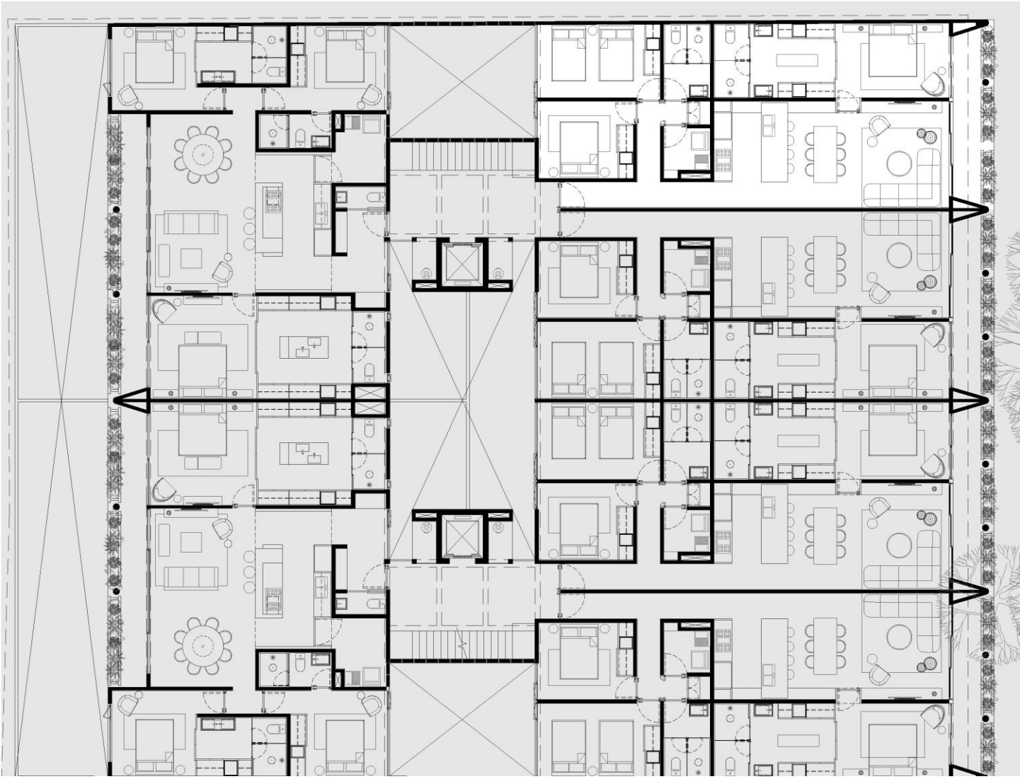
CUARTO NIVEL
