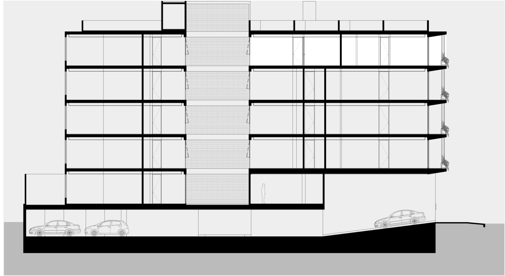
CORTE ESQUEMÁTICO
