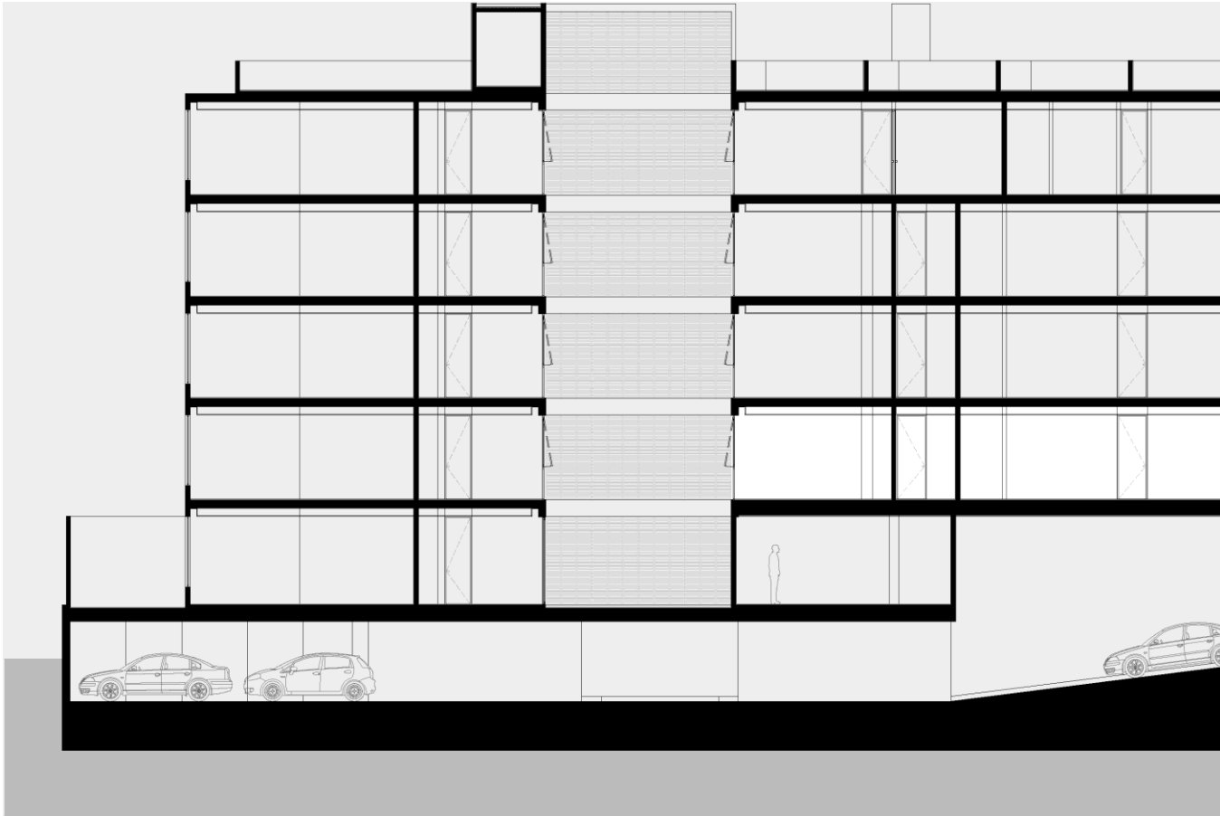
CORTE ESQUEMÁTICO
