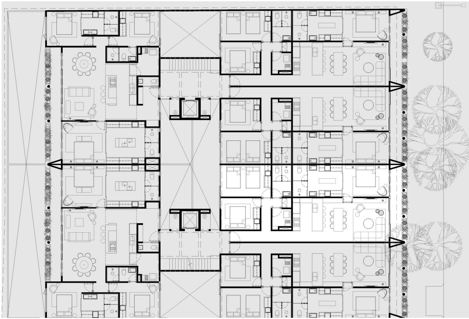
CUARTO NIVEL
