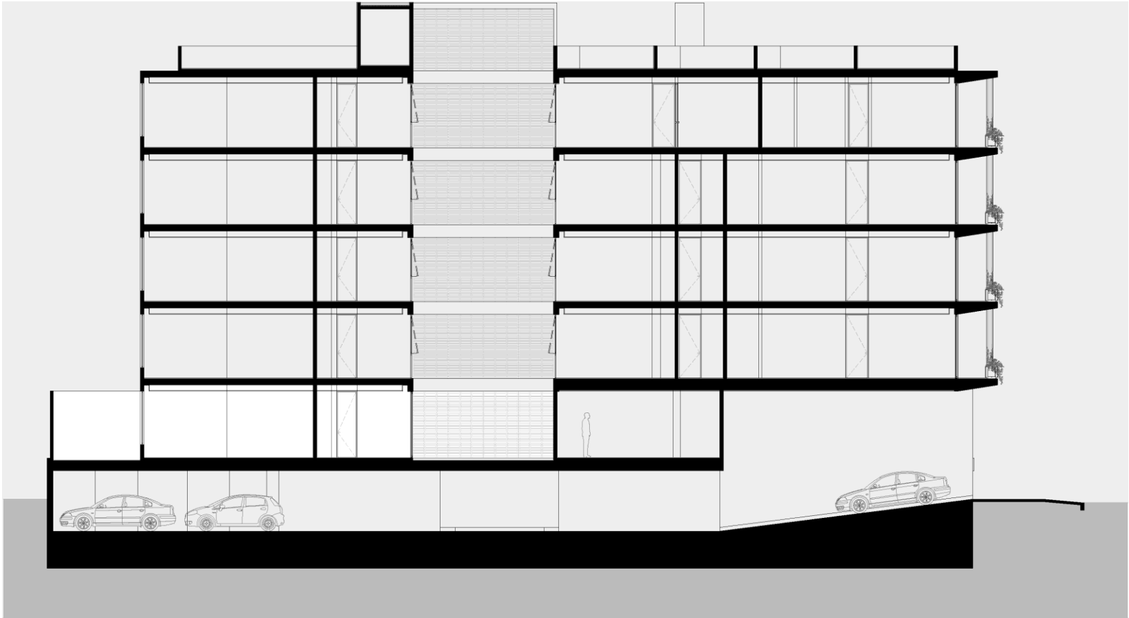
CORTE ESQUEMÁTICO
