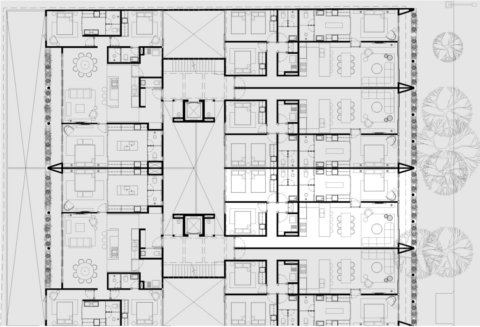
TERCER NIVEL
