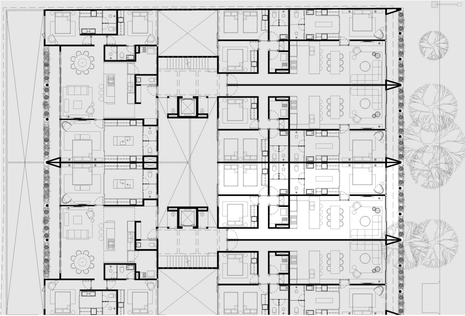
SEGUNDO NIVEL
