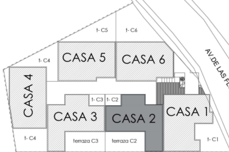
PLANTA CONJUNTO
