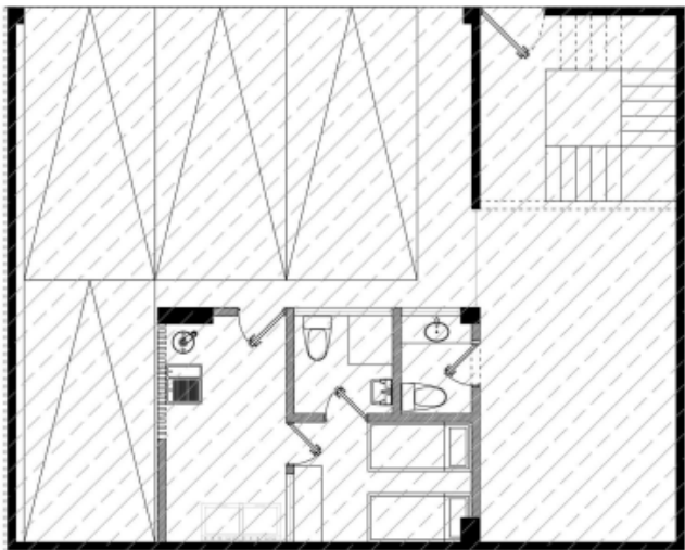
SEMI-SÓTANO Área 123m 2
